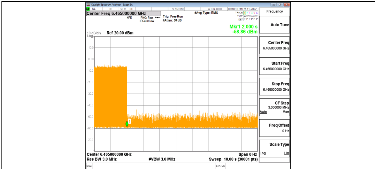
11AX80MIMO_Ant1_6465_Center_6465_10
