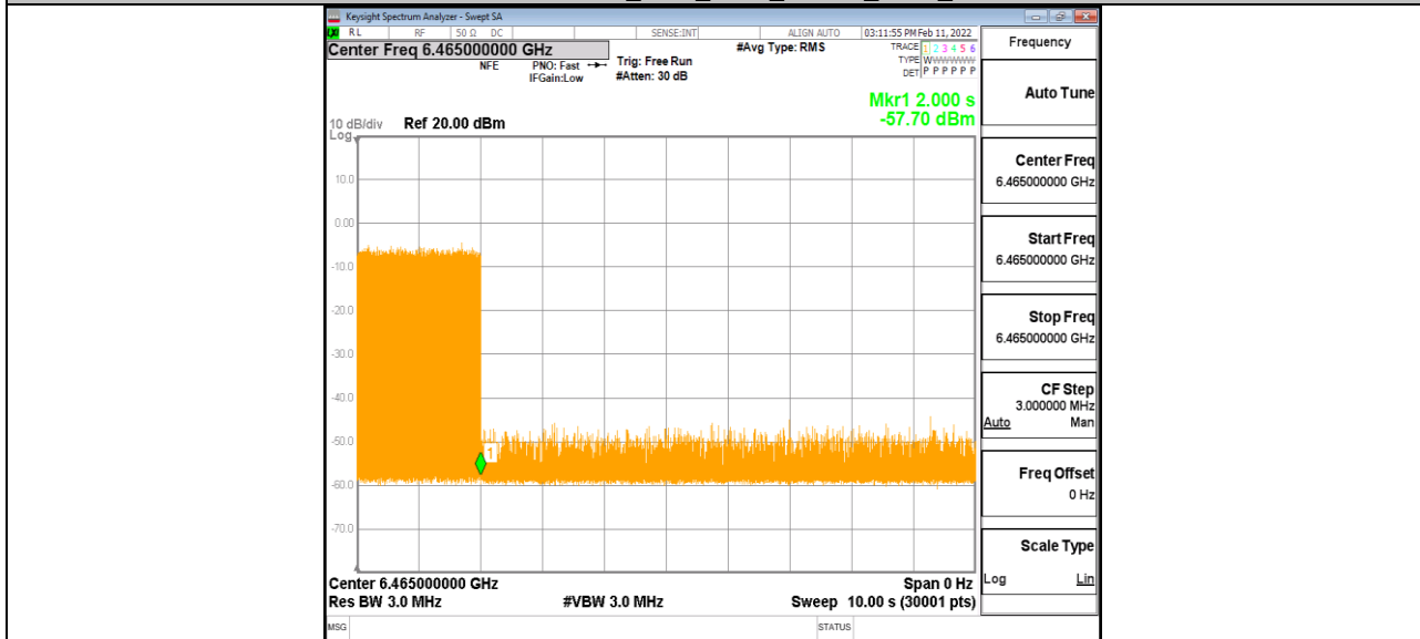
11AX80MIMO_Ant1_6465_Center_6465_5
