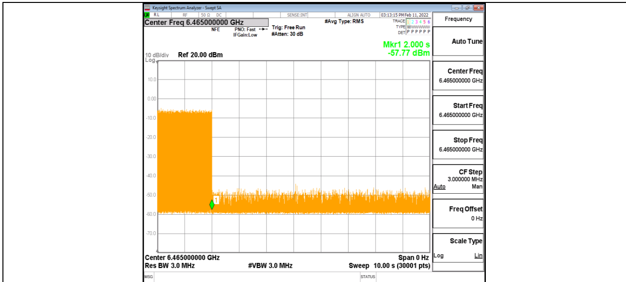
11AX80MIMO_Ant1_6465_Center_6465_6
