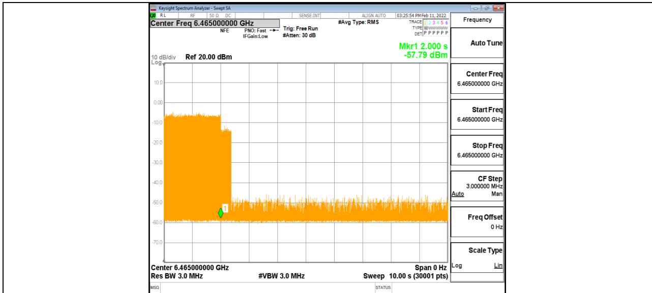
11AX80MIMO_Ant1_6465_Low_6500_6
