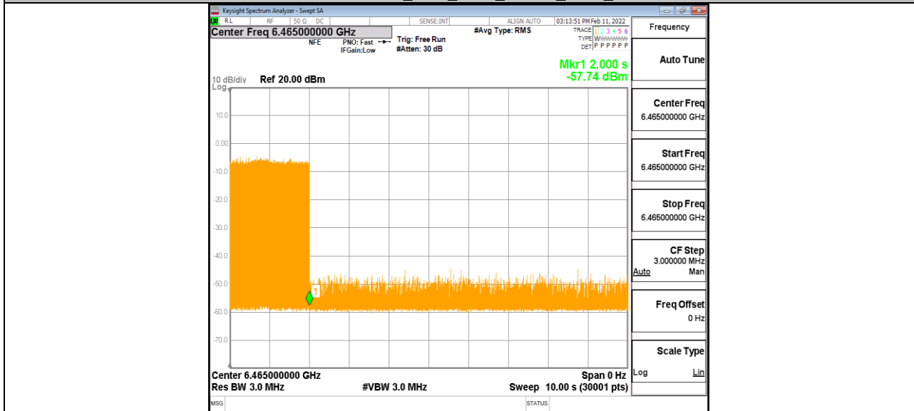
11AX80MIMO_Ant1_6465_Center_6465_7
