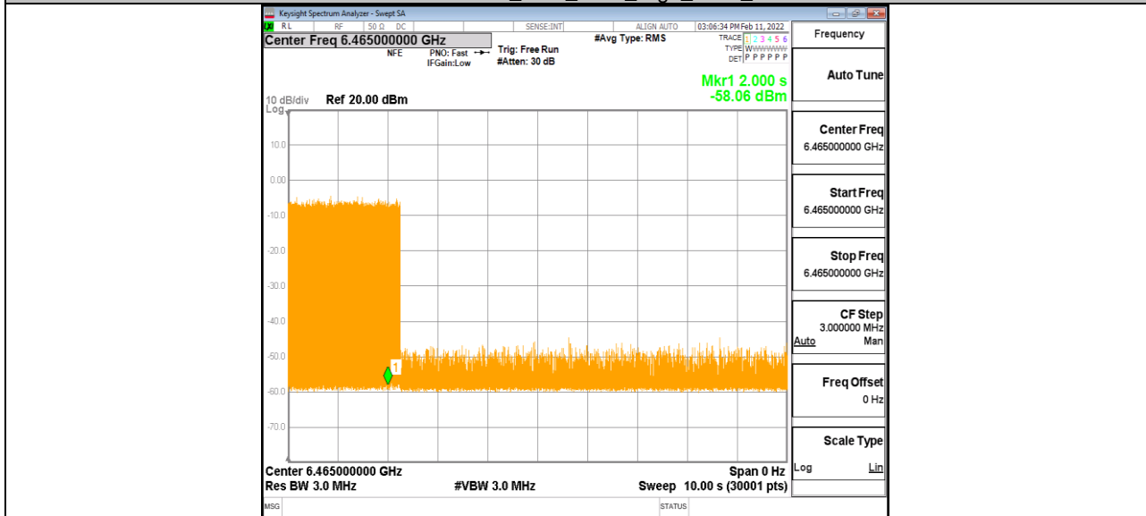
11AX80MIMO_Ant1_6465_Center_6465_1
