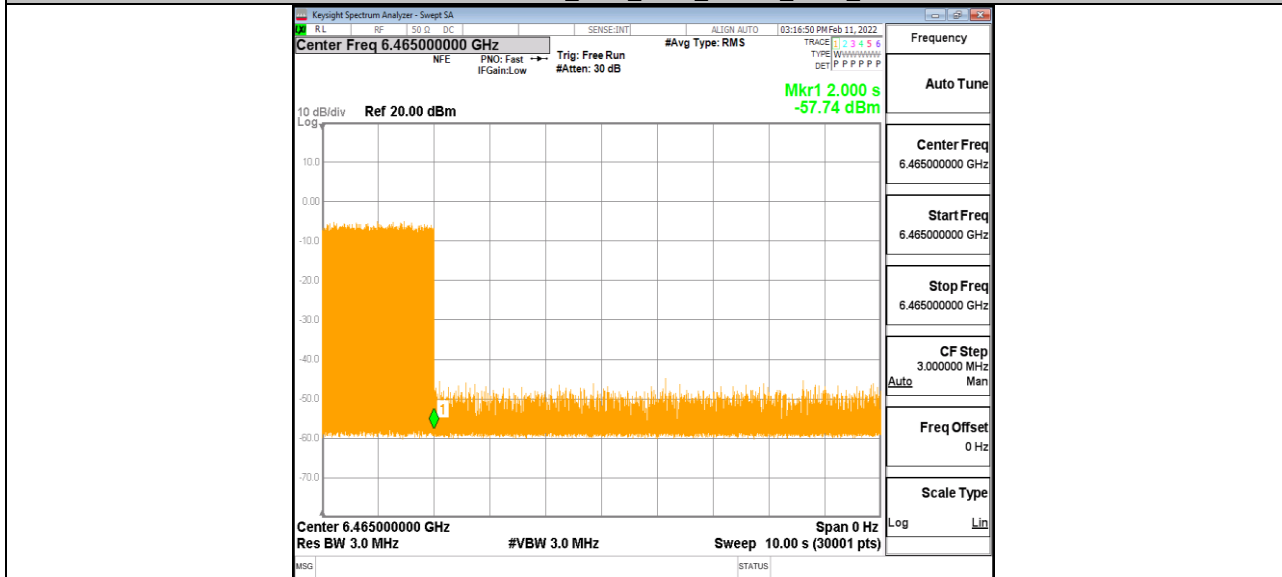
11AX80MIMO_Ant1_6465_Center_6465_9
