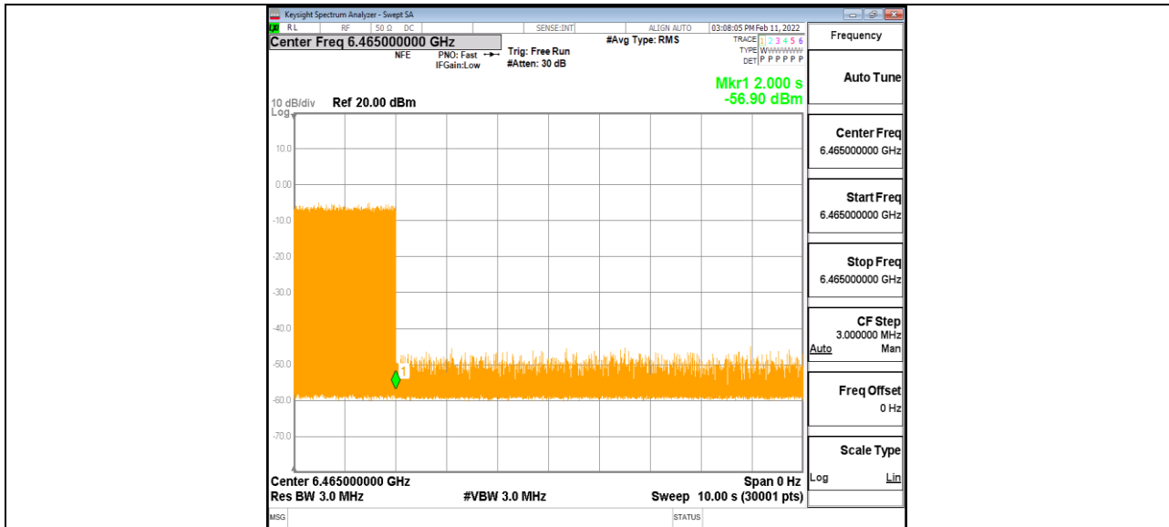
11AX80MIMO_Ant1_6465_Center_6465_2
