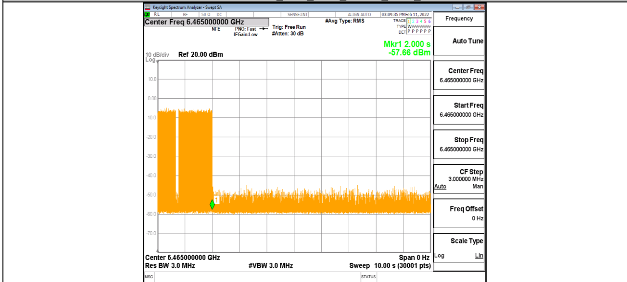
11AX80MIMO_Ant1_6465_Center_6465_3
