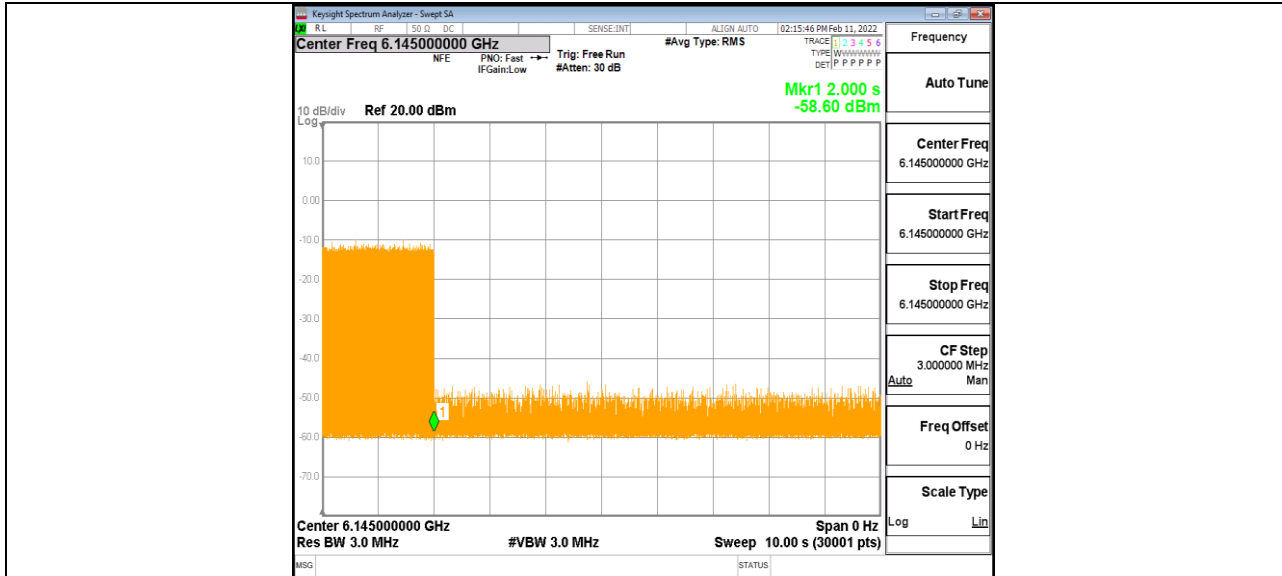
11AX80MIMO_Ant1_6145_Center_6145_4
