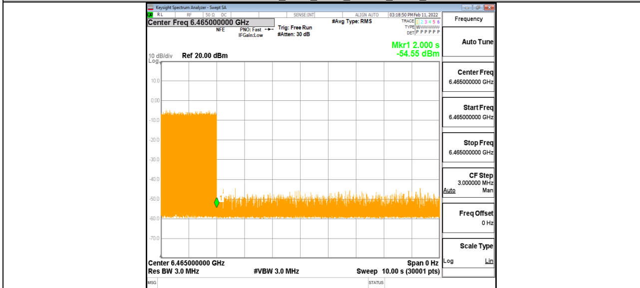
11AX80MIMO_Ant1_6465_Low_6500_1
