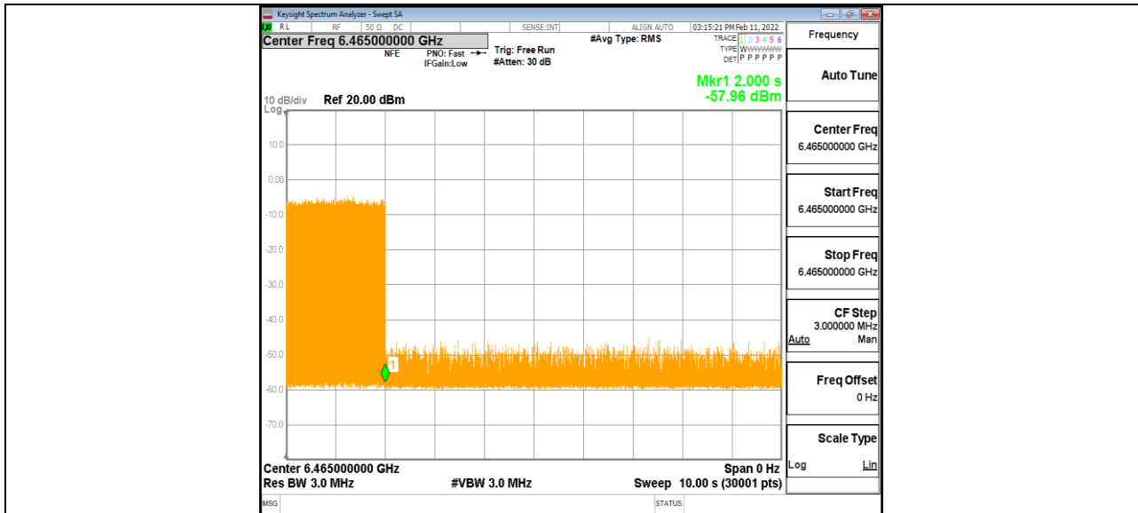
11AX80MIMO_Ant1_6465_Center_6465_8
