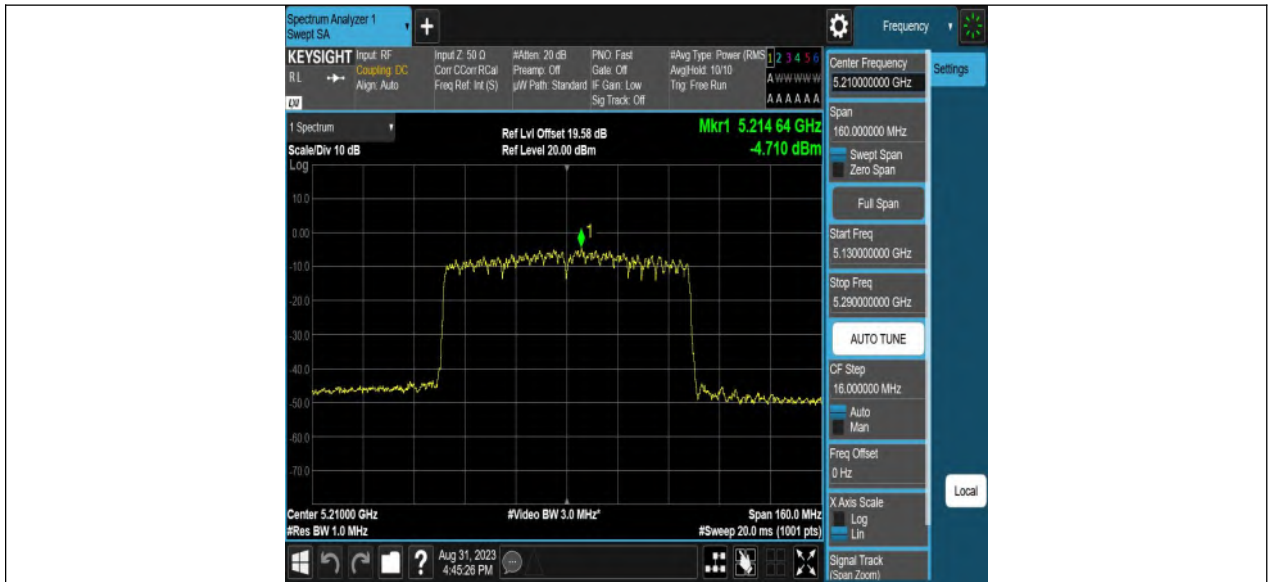
11AC80MIMO_Ant2_5210
