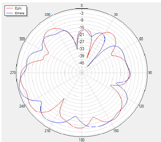
Theta=90 freq=2500MHz
