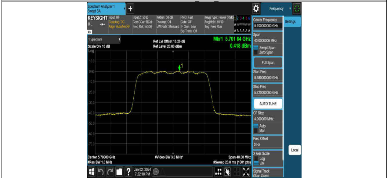
11N20MIMO Ant2 5700
