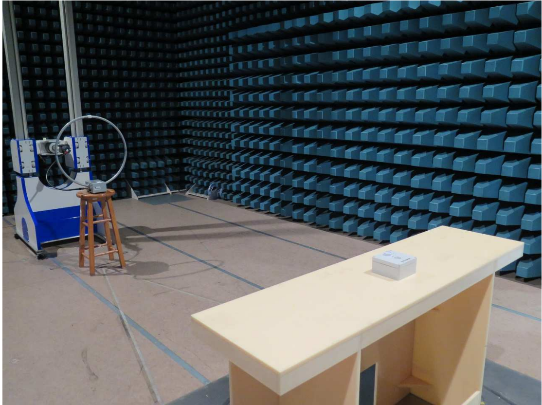
9kHz – 30MHz
