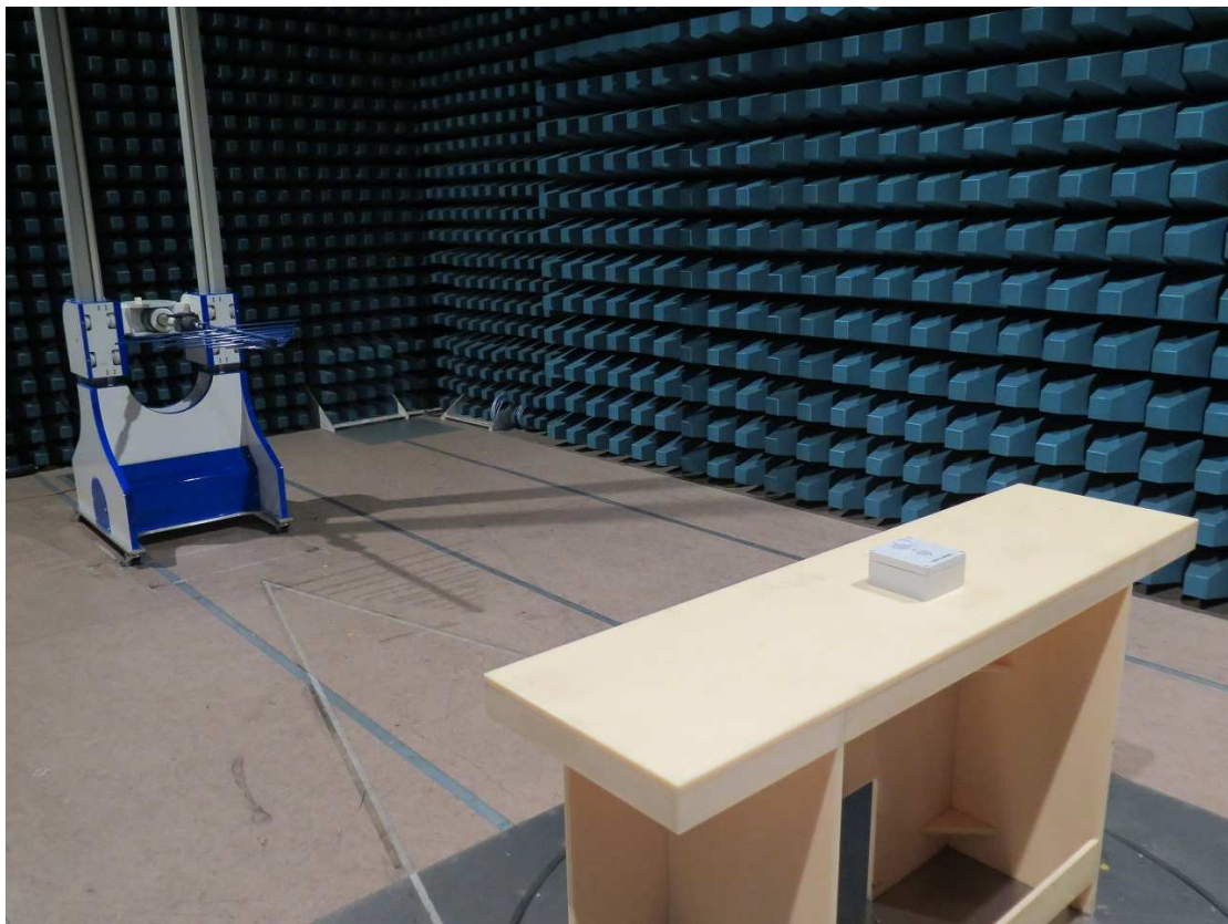
200MHz – 1GHz
