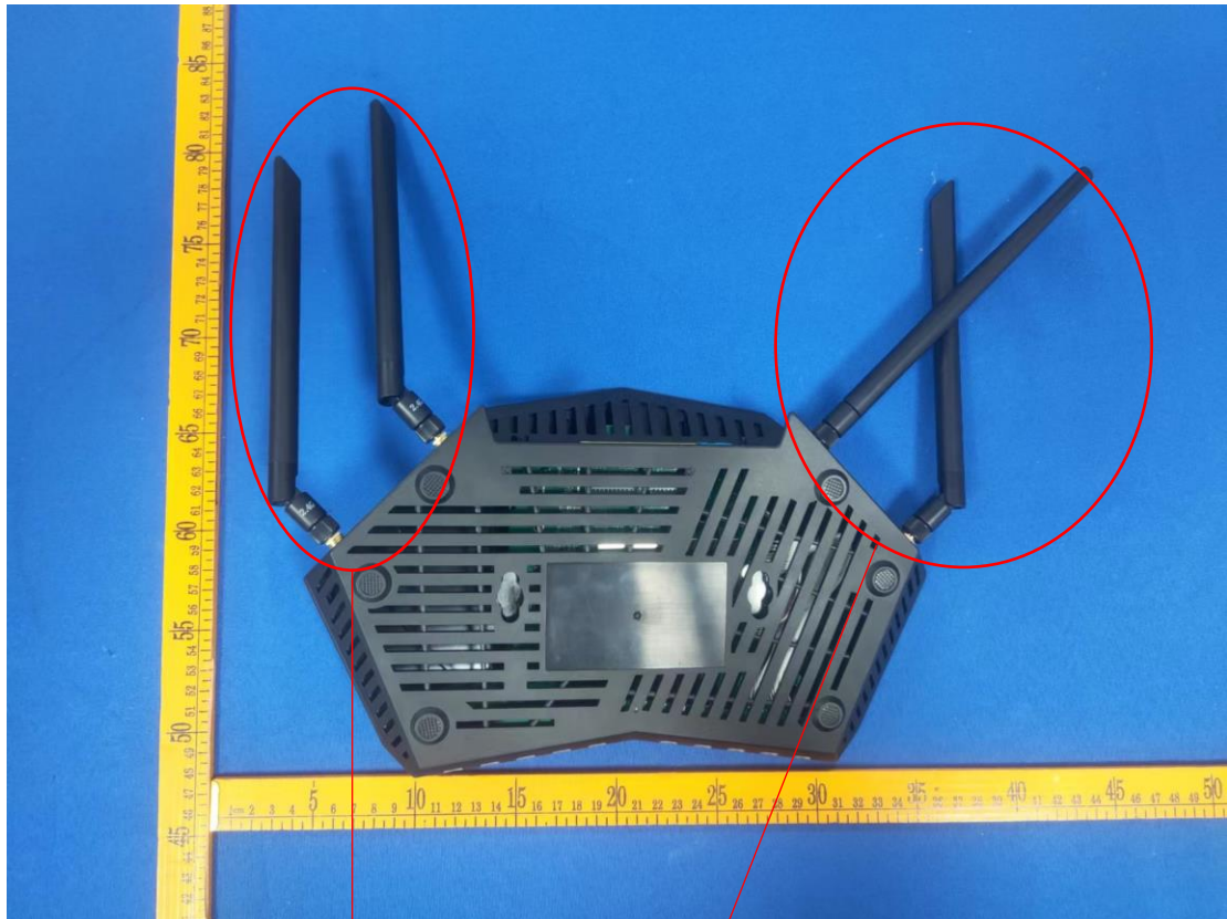
2.4G antenna
