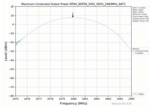
8DPSK_2480MHz_3DH5_SISO_ANT1
