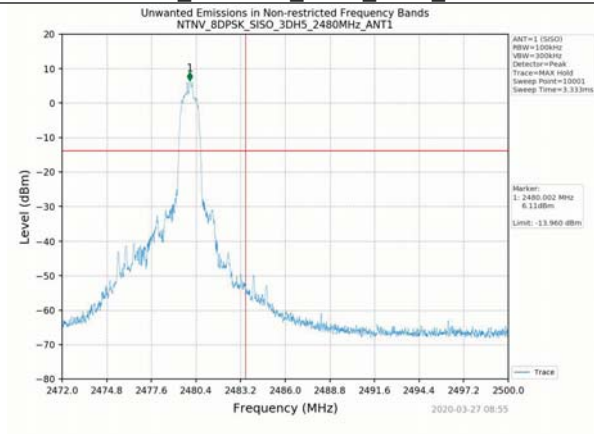
8DPSK_2480MHz_3DH5_SISO_ANT1
