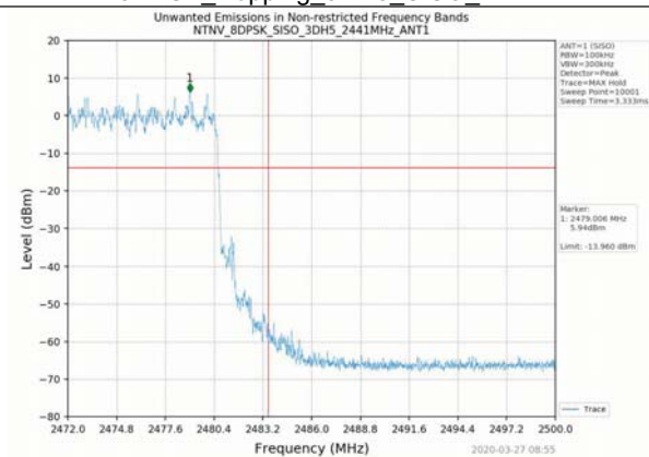
8DPSK_Hopping_3DH5_SISO_ANT1
