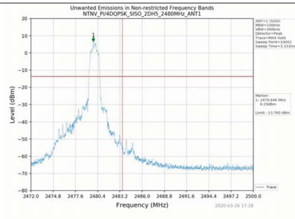
Pi/4DQPSK_2480MHz_2DH5_SISO_ANT1
