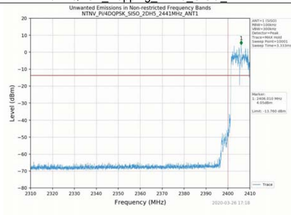
Pi/4DQPSK_Hopping_2DH5_SISO_ANT1
