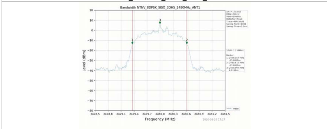
8DPSK_2480MHz_3DH5_SISO_ANT1
