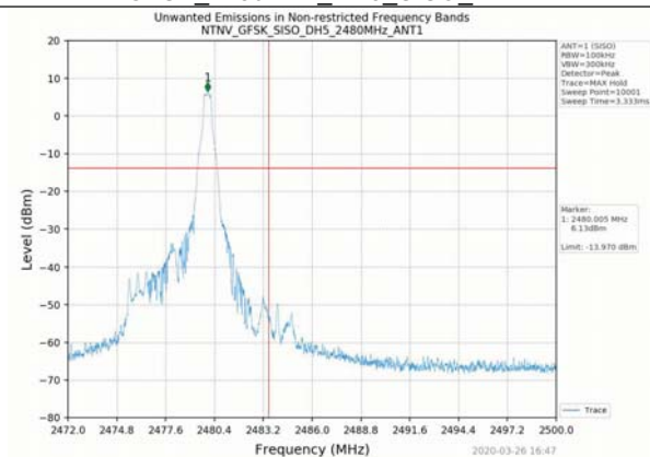
GFSK_2480MHz_DH5_SISO_ANT1
