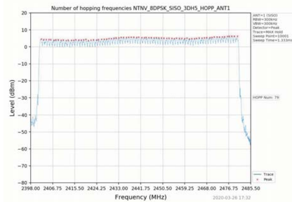
8DPSK_Hopping_3DH5_SISO_ANT1
