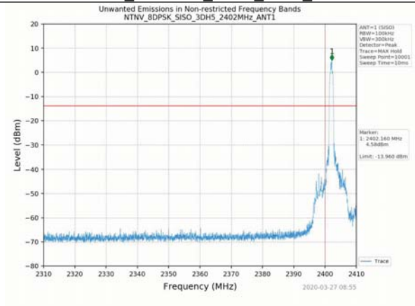
8DPSK_2402MHz_3DH5_SISO_ANT1
