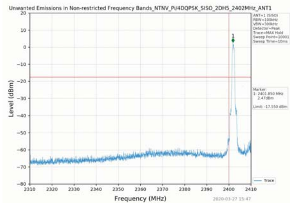
Pi/4DQPSK_2402MHz_2DH5_SISO_ANT1
