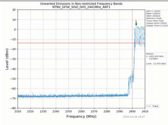
GFSK_Hopping_DH5_SISO_ANT1
