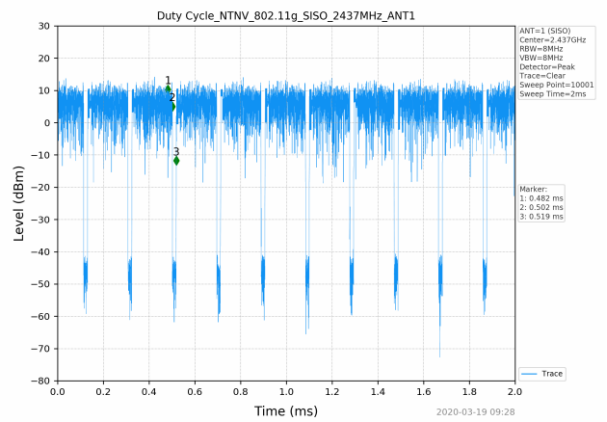
802.11g_2437MHz_SISO_ANT1
