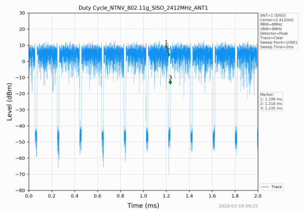
802.11g_2412MHz_SISO_ANT1
