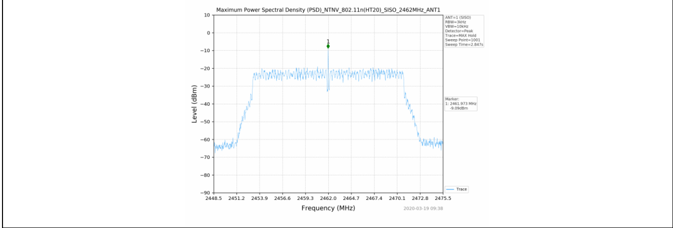
802.11n(HT20)_2462MHz_SISO_ANT1
