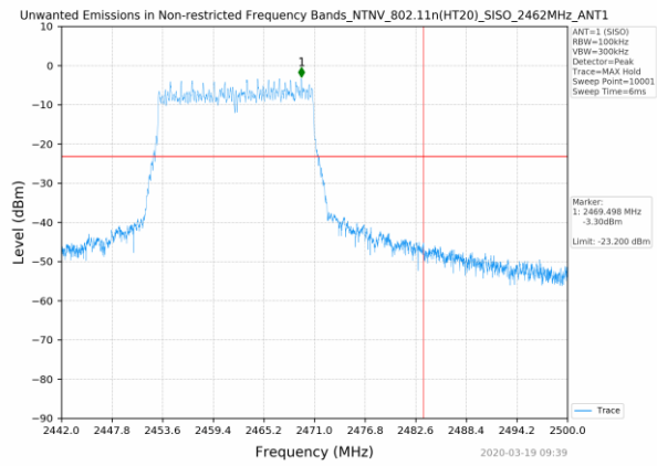
802.11n(HT20)_2462MHz_SISO_ANT1
