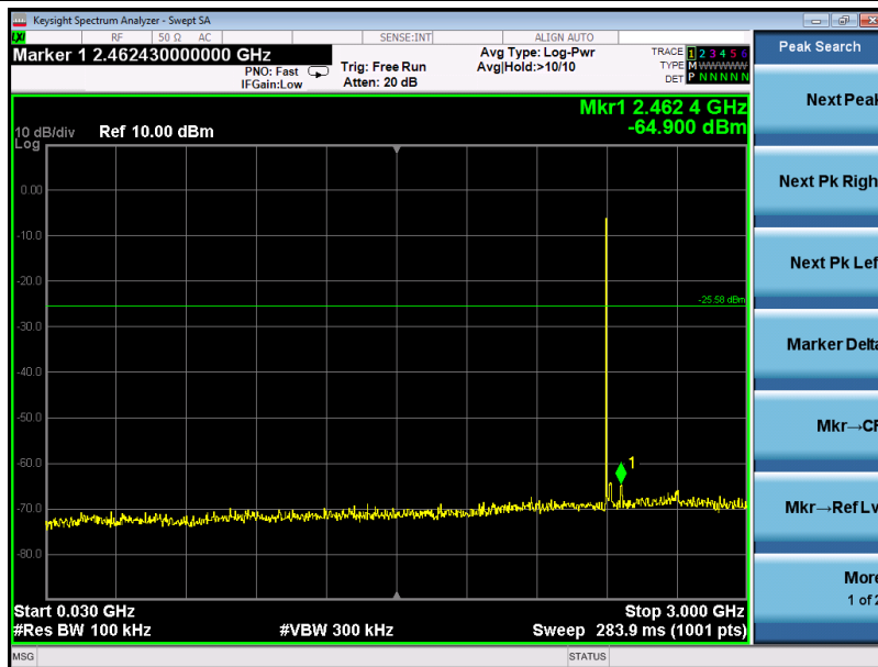
30MHz~3GHz
