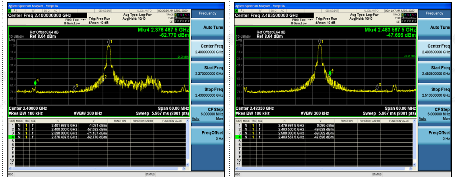
Left Band edge hopping off
