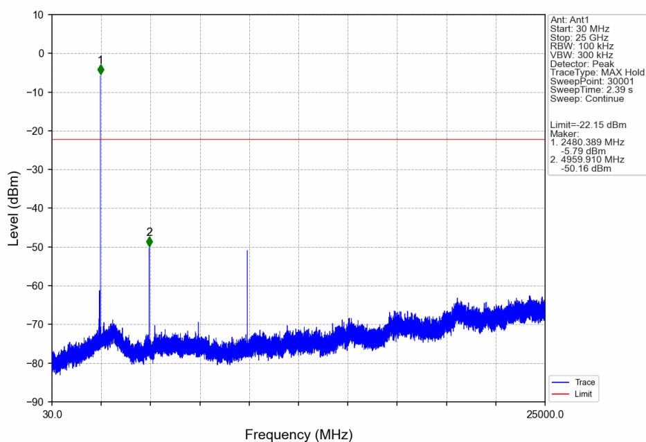
GFSK DH5 HOPP Ant1_NTNV
