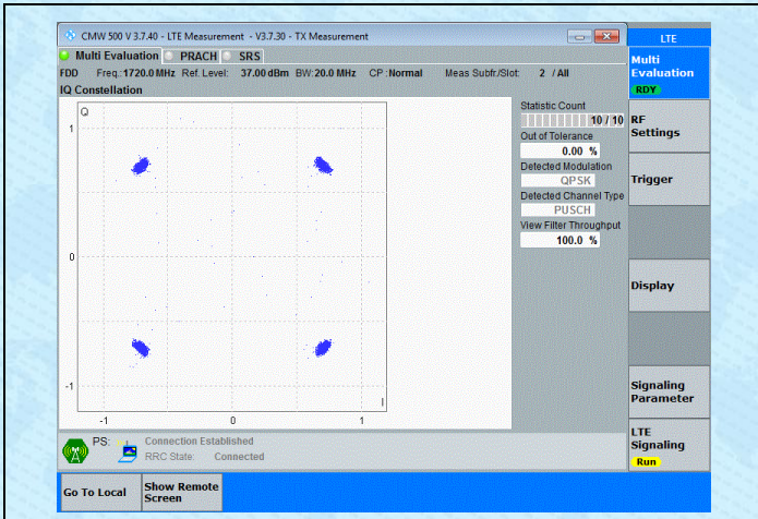
Band4-20MHz-QPSK-20050-100RB#0-PASS
