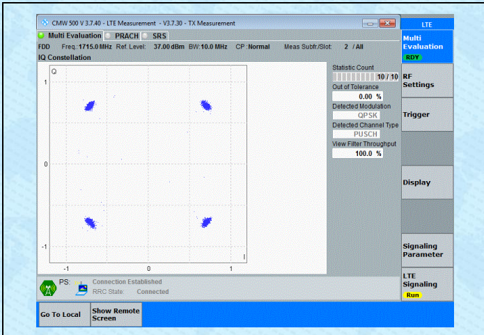
Band4-10MHz-QPSK-20000-50RB#0-PASS
