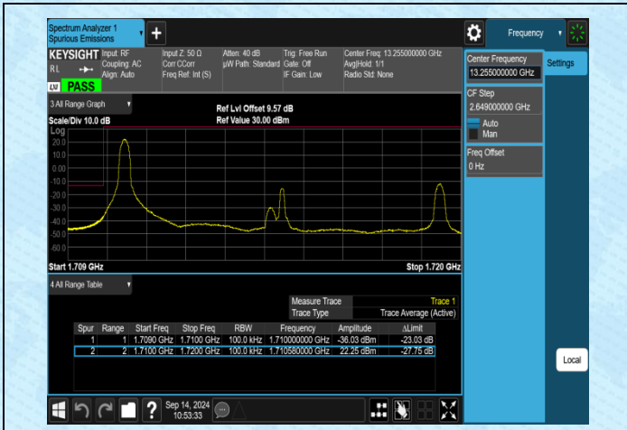
Band4-10MHz-QPSK-20000-1RB#0-PASS
