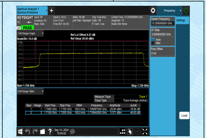
Band4-10MHz-QPSK-20000-50RB#0-PASS
