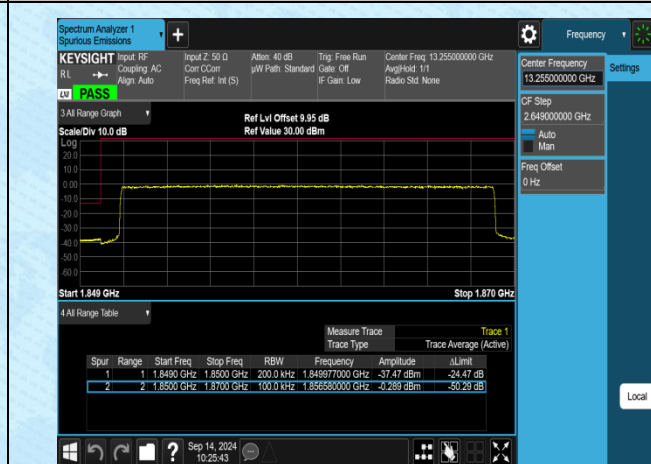
Band2-20MHz-QPSK-18700-100RB#0-PASS
