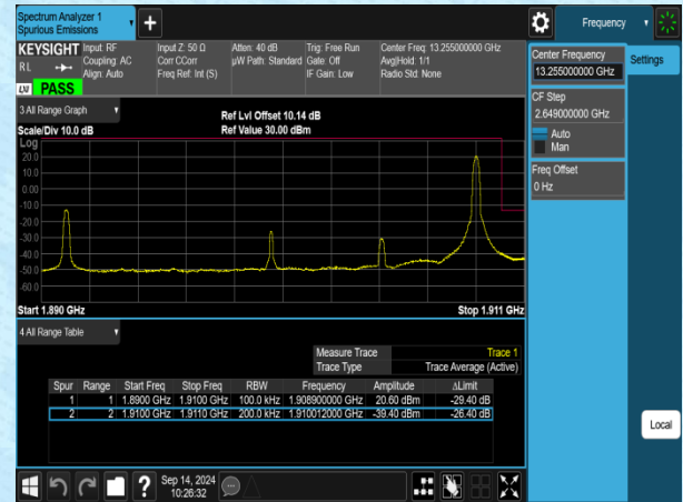
Band2-20MHz-16QAM-19100-1RB#99-PASS
