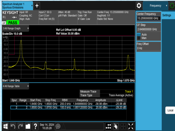
Band2-20MHz-16QAM-18700-1RB#0-PASS
