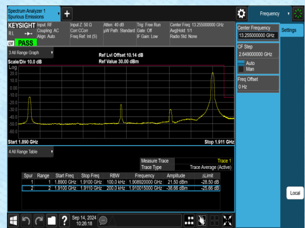
Band2-20MHz-QPSK-19100-1RB#99-PASS
