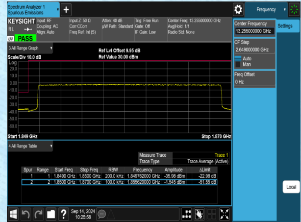
Band2-20MHz-16QAM-18700-100RB#0-PASS
