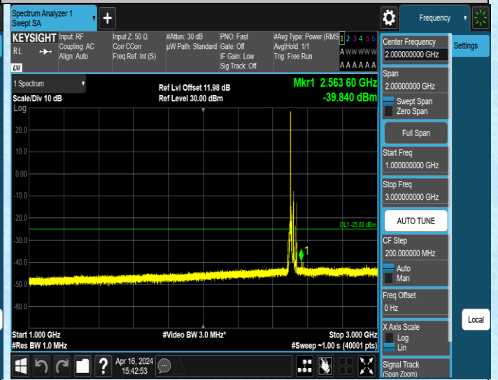
Band7_20MHz_QPSK_20850_1RB#0_1000~3000_1000~3000 0
