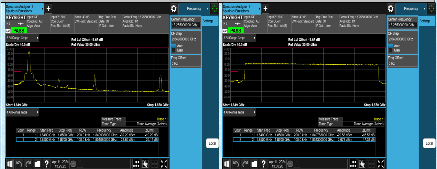
Band2_20MHz_QPSK_18700_1RB#0
