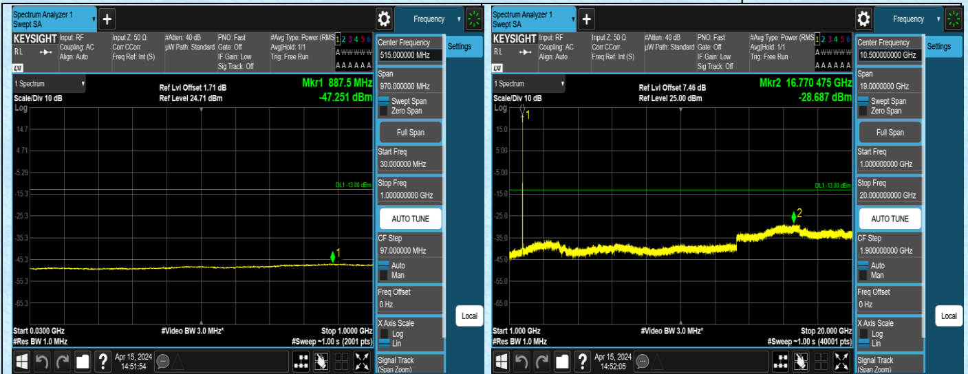
Band4-1413-30~1000MHz-PASS
