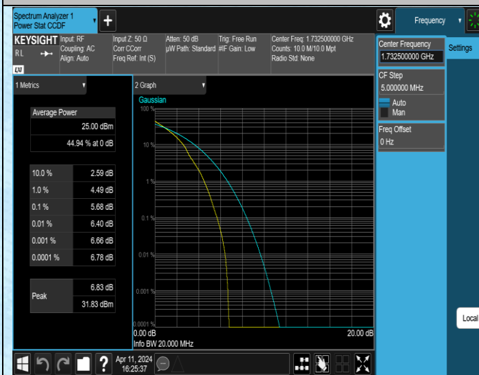
Band4-20MHz-QPSK-20175-1RB#0-PASS
