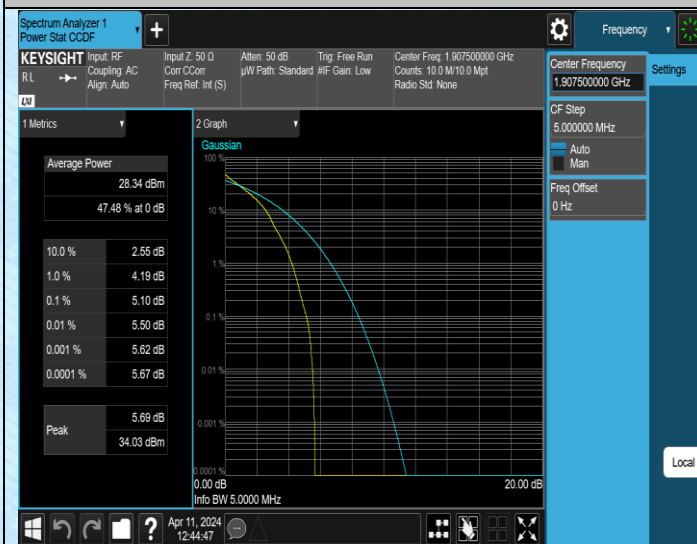
Band2-5MHz-QPSK-19175-1RB#0-PASS
