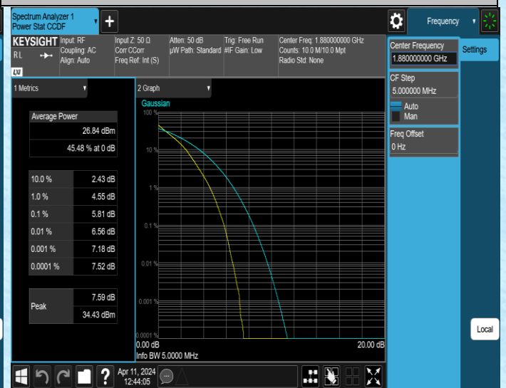
Band2-5MHz-QPSK-18900-25RB#0-PASS
