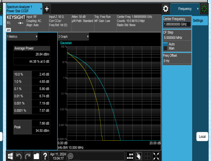
Band2-10MHz-QPSK-18900-50RB#0-PASS
