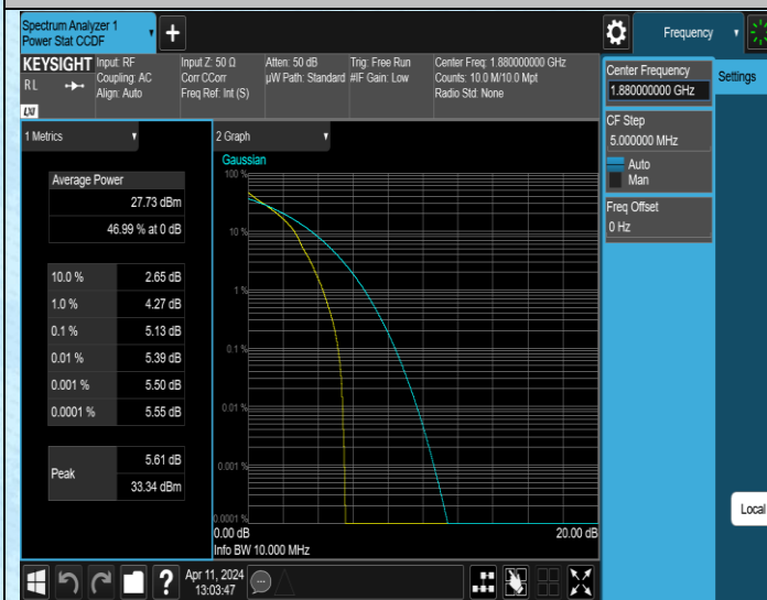
Band2-10MHz-QPSK-18900-1RB#0-PASS
