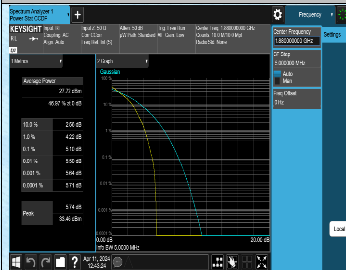
Band2-5MHz-QPSK-18900-1RB#0-PASS
