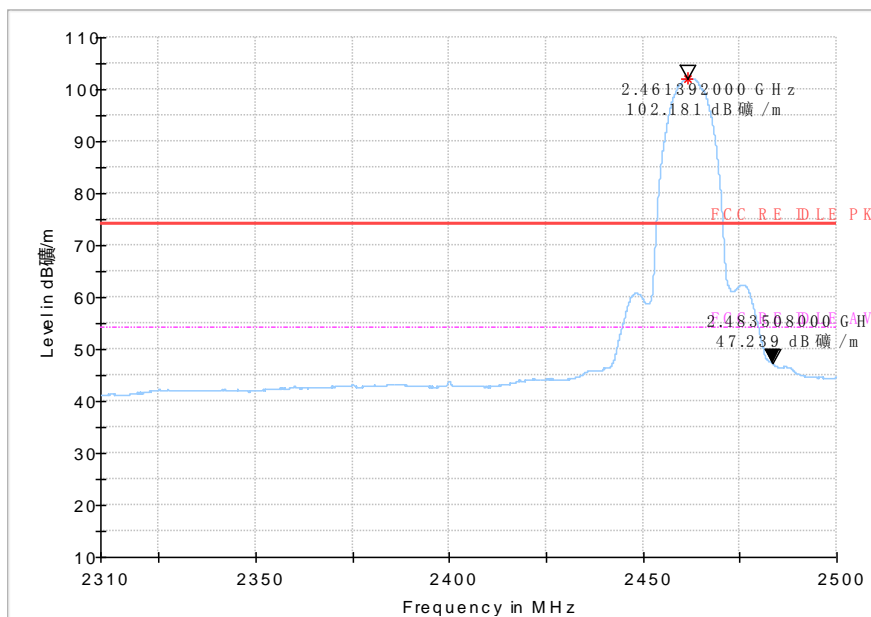
AV detector
