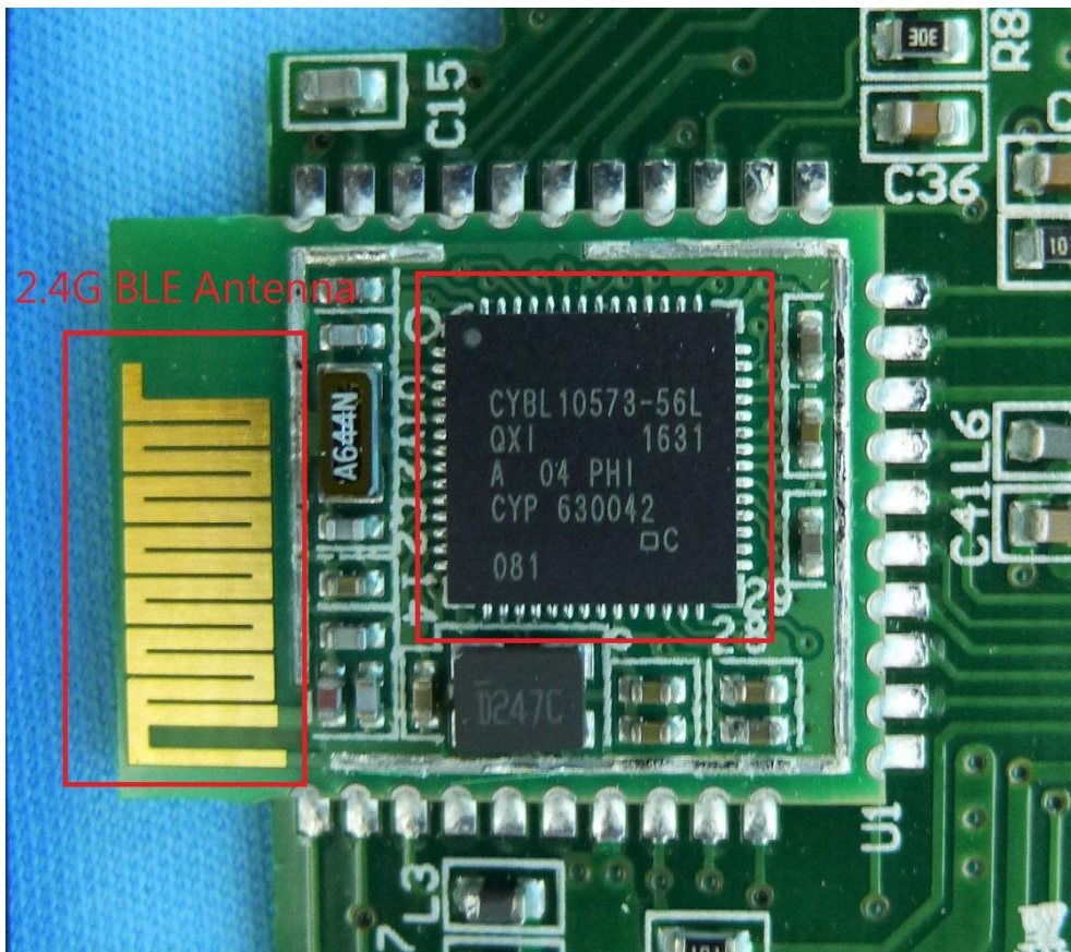
(14) EUT Photo
