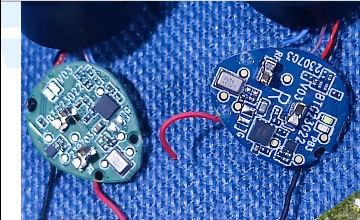
EUT Photo
