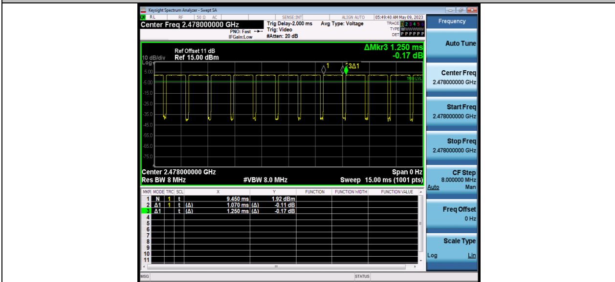
BLE_2M_Ant1_2478
