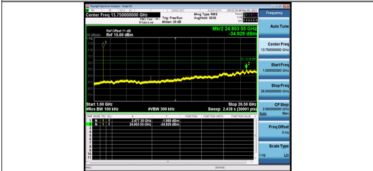
BLE_2M_Ant1_2478_1000~26500
