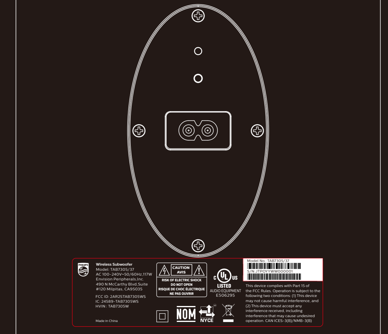
Subwoofer Back
