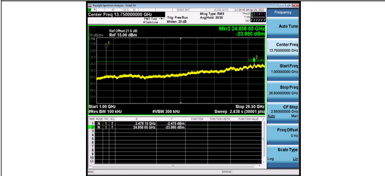
BLE_2M_Ant1_2478_1000~26500
