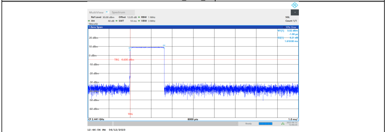
DH3_Ant1_Hop
