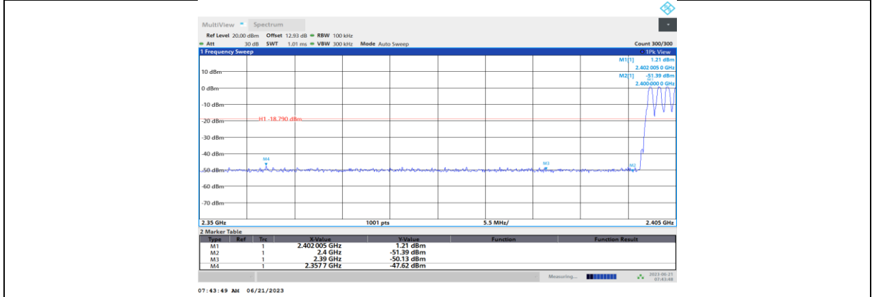
DH5_Ant1_Low_Hop_2402
