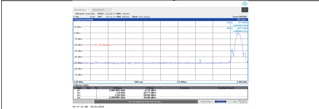
BLE_2M_Ant1_Low_2402
