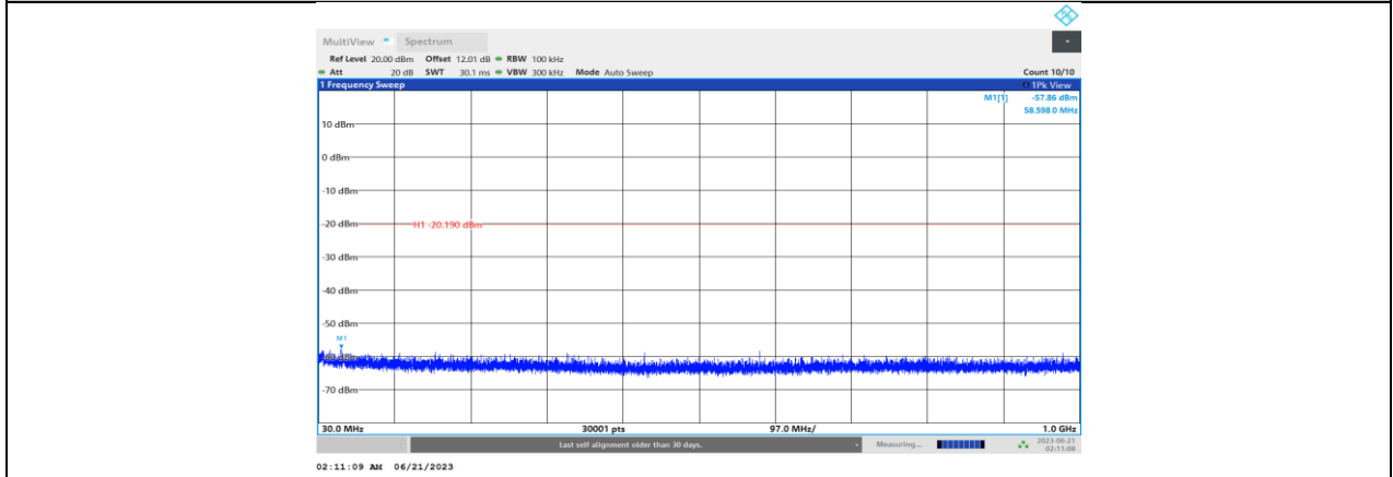
BLE_2M_Ant1_2480_30~1000
