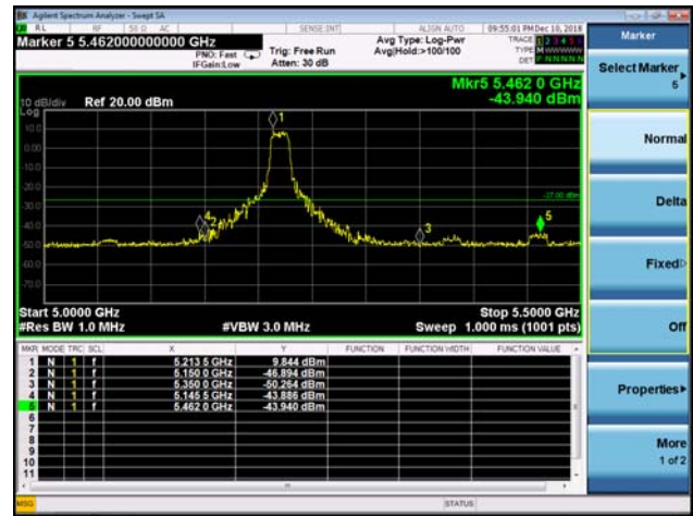
ANTB (5.2 GHz) Band Edge
