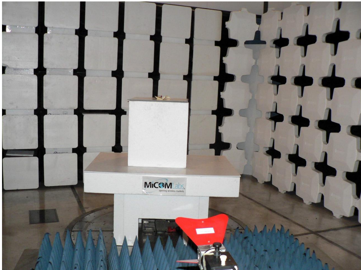
SHOO03 TX Spurious Integral 1-18GHz
