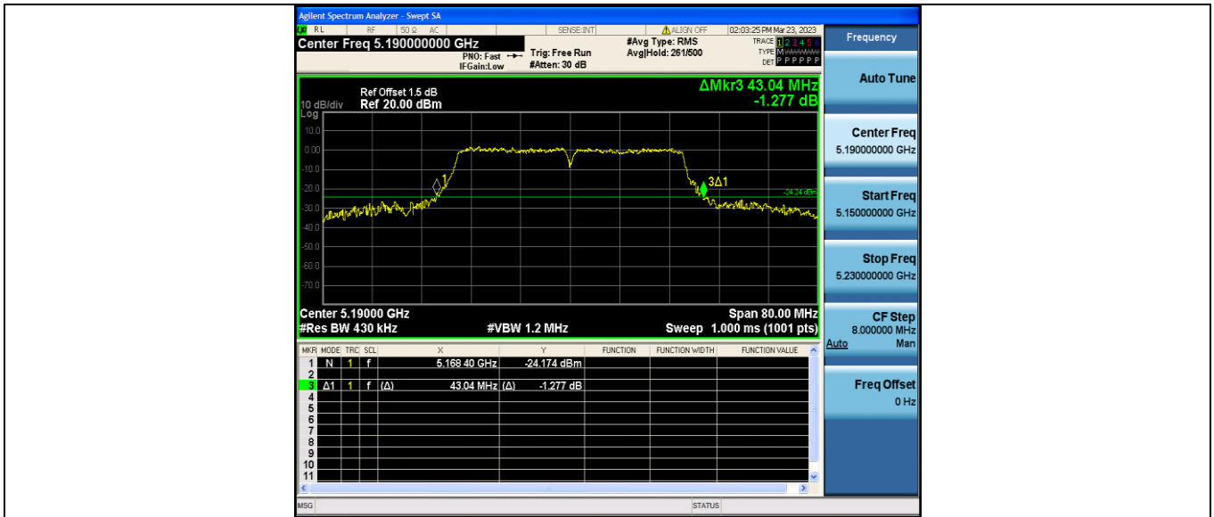
11N40MIMO_Ant2_5190
