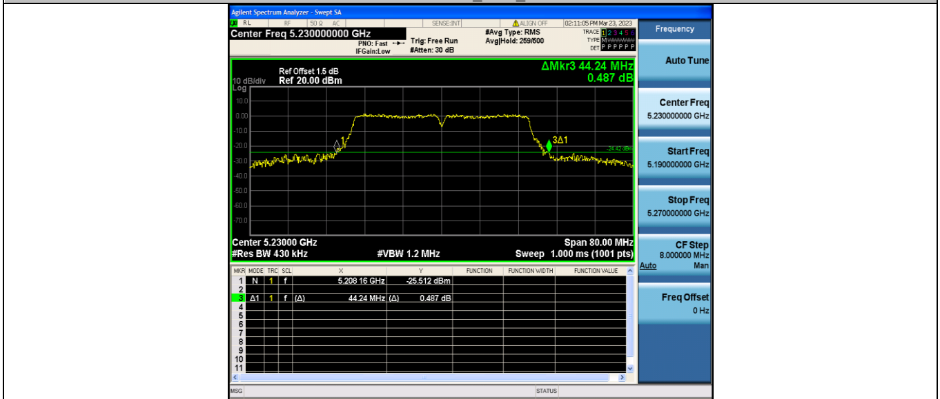
11N40MIMO_Ant2_5230
