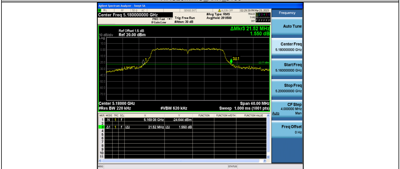
11AC20MIMO_Ant2_5180
