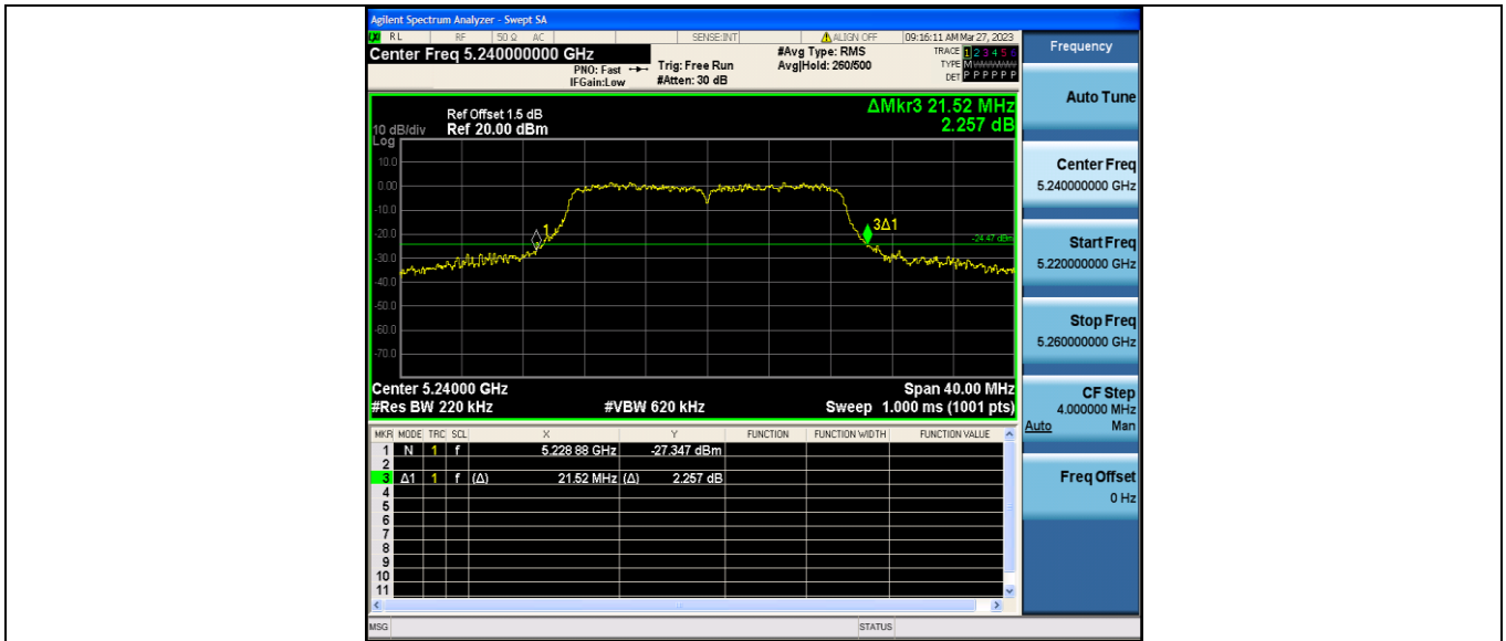
11AC20MIMO_Ant2_5240
