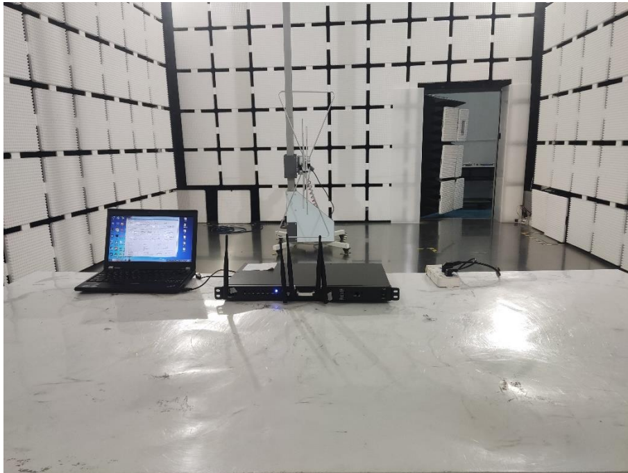
30-1000MHz
