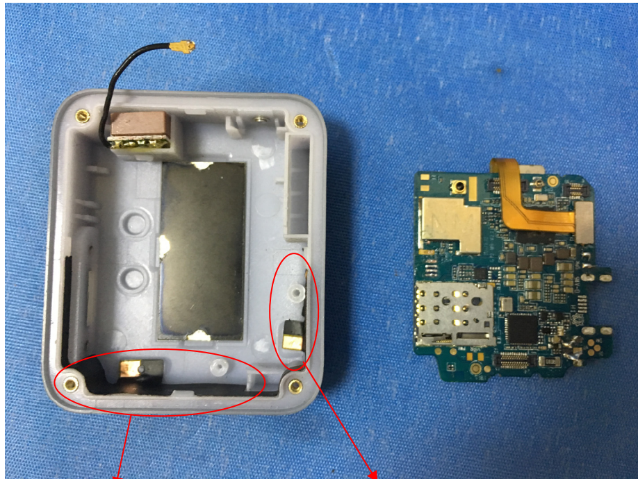
BT/WIFI/BLE ANT.
