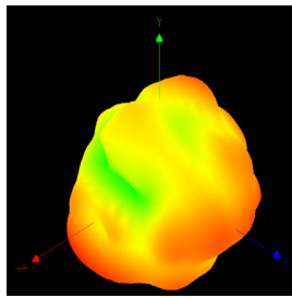
BT 天线方向图
