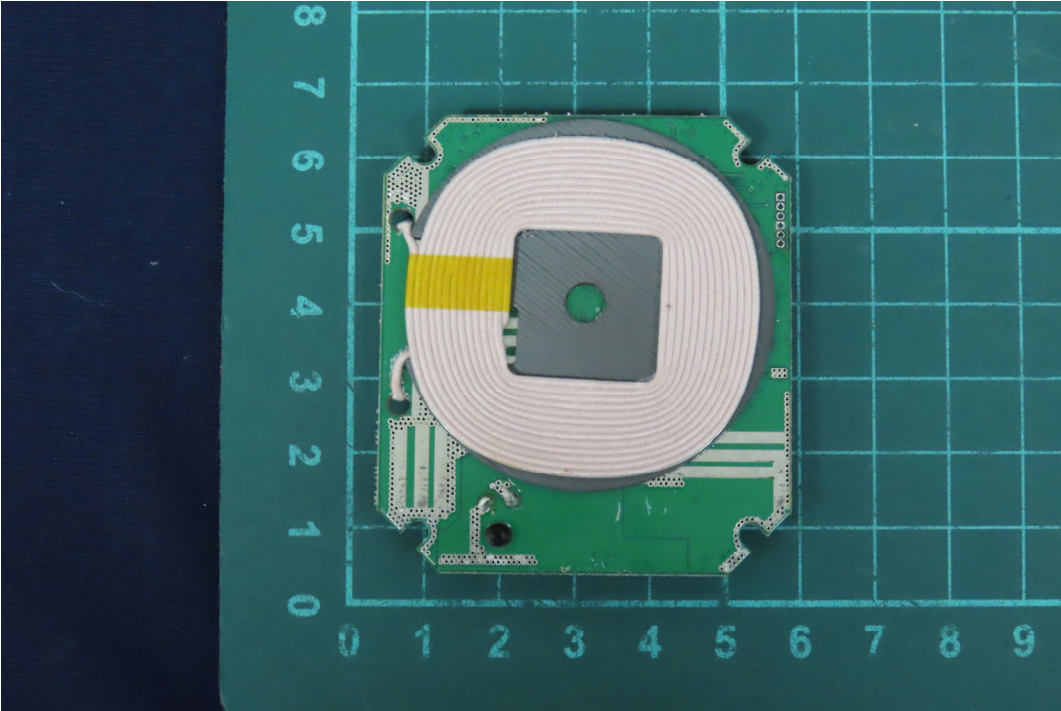
(4) EUT Photo (Antenna)
