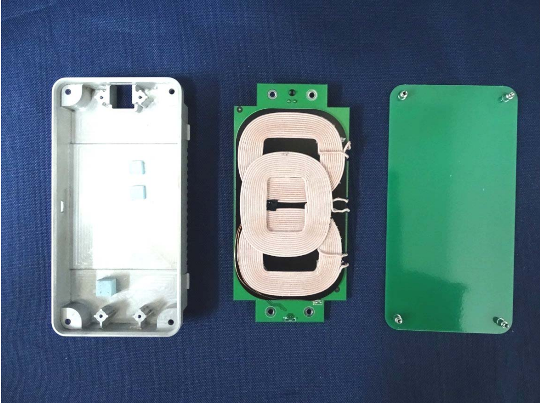
(3) EUT Photo
