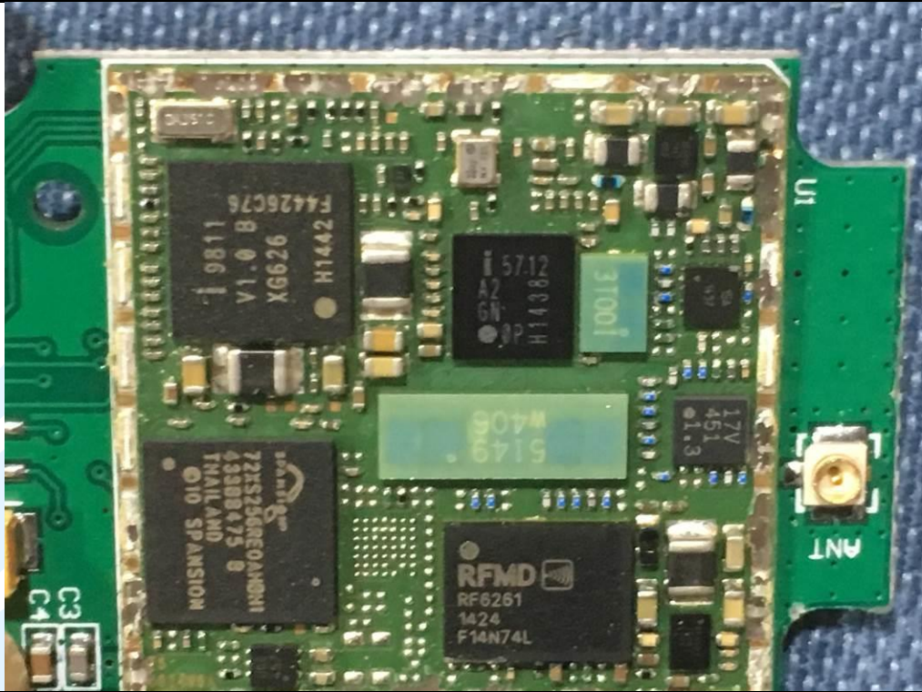
EUT Photo (WCDMA module)
