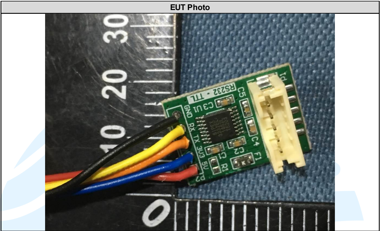
EUT Photo (WCDMA module)
