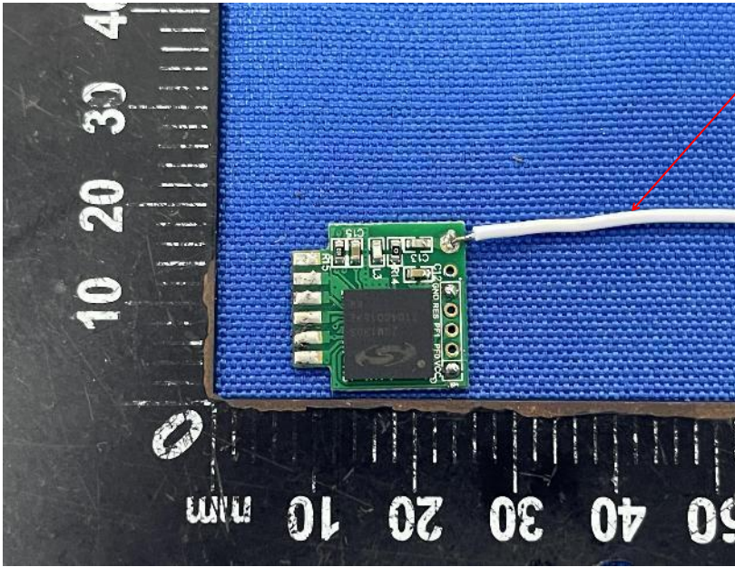
Antenna
