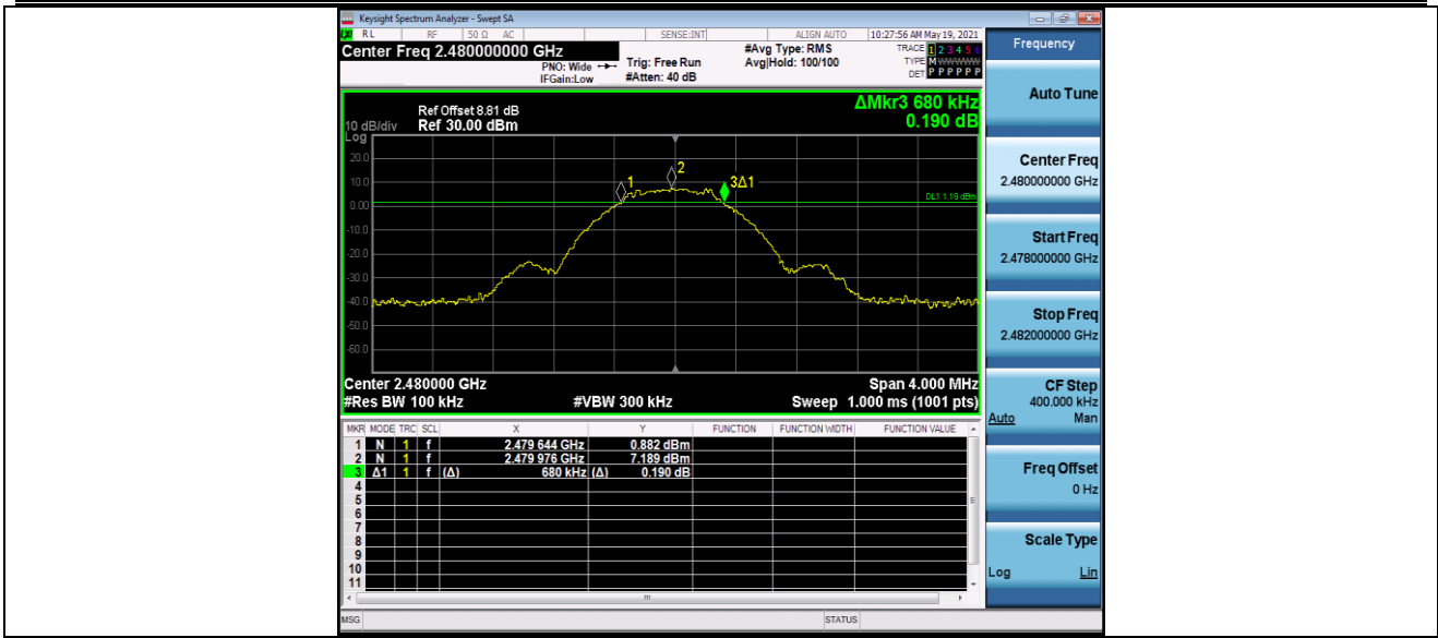
BLE_BT4.0_Ant1_2480
