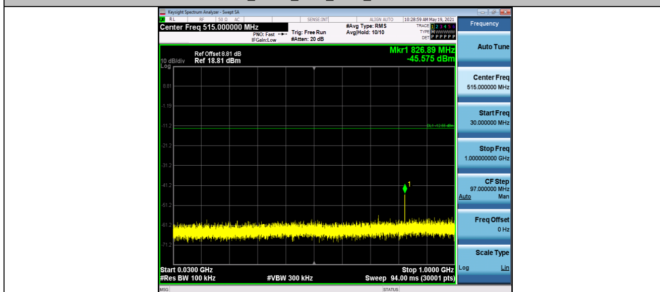
BLE_BT4.0_Ant1_2480_30~1000
