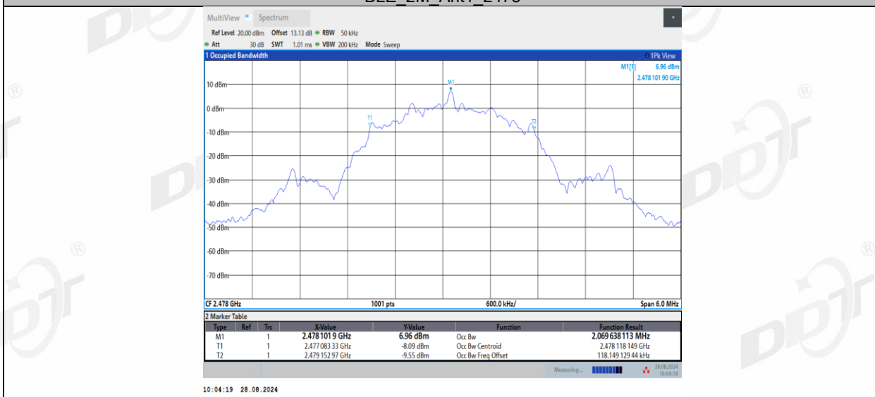
BLE_2M_Ant1_2478
