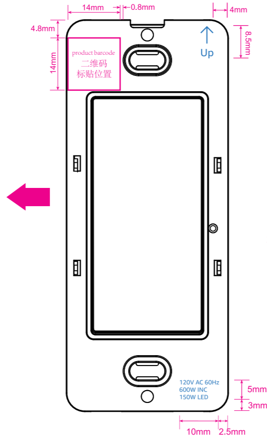
Switch 正面(镭雕)
