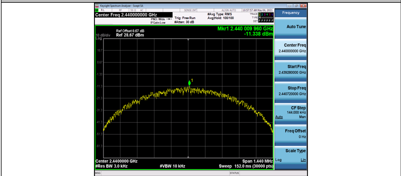
BLE_BT4.2_Ant1_2440
