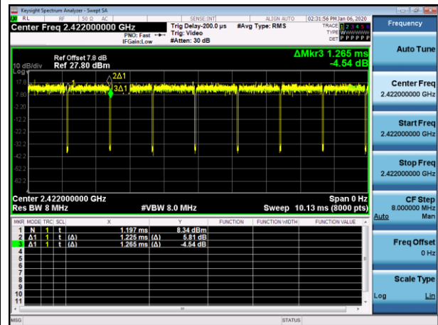
802.11n HT40
