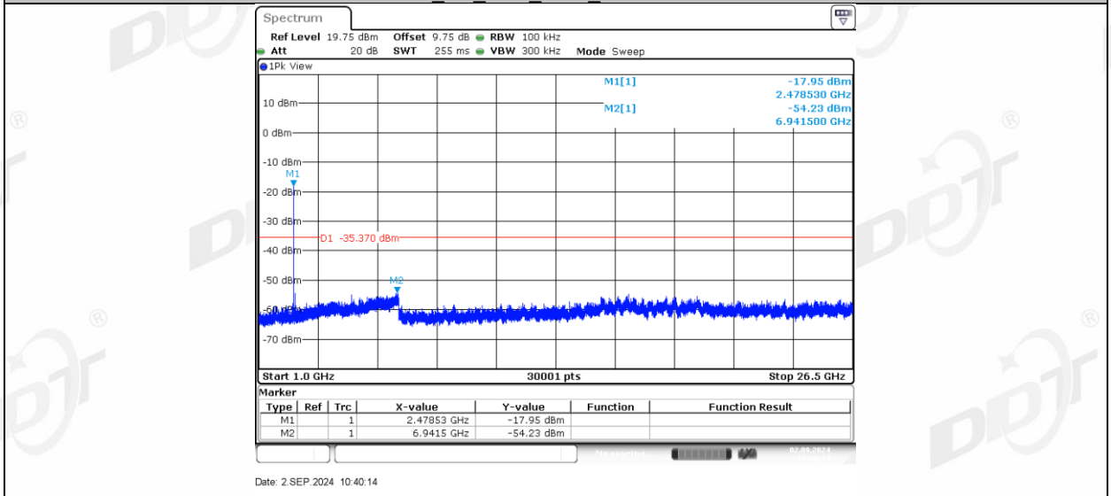
BLE_2M_Ant1_2478_1000~26500
