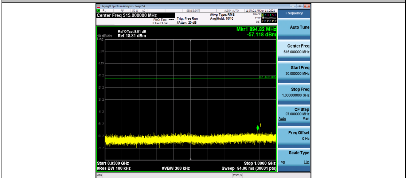
BLE_BT4.2_Ant1_2480_30~1000
