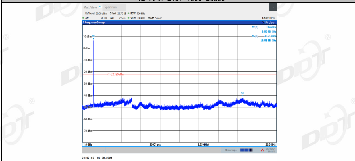
11B_Ant1_2462_0~Reference
