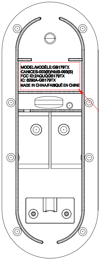
18000179下盖 刻字镶块位置示意图0809
