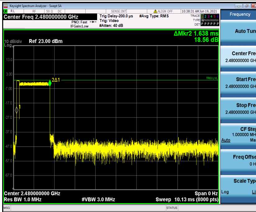
2DH3_Ant1_Hop_2480
