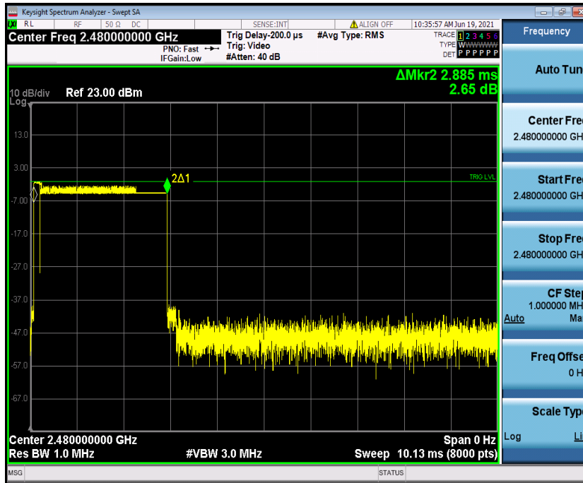
2DH5_Ant1_Hop_2480
