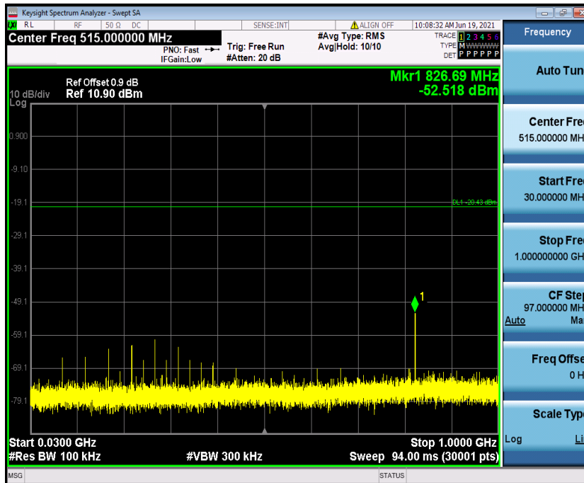
DH5_Ant1_2480_30~1000
