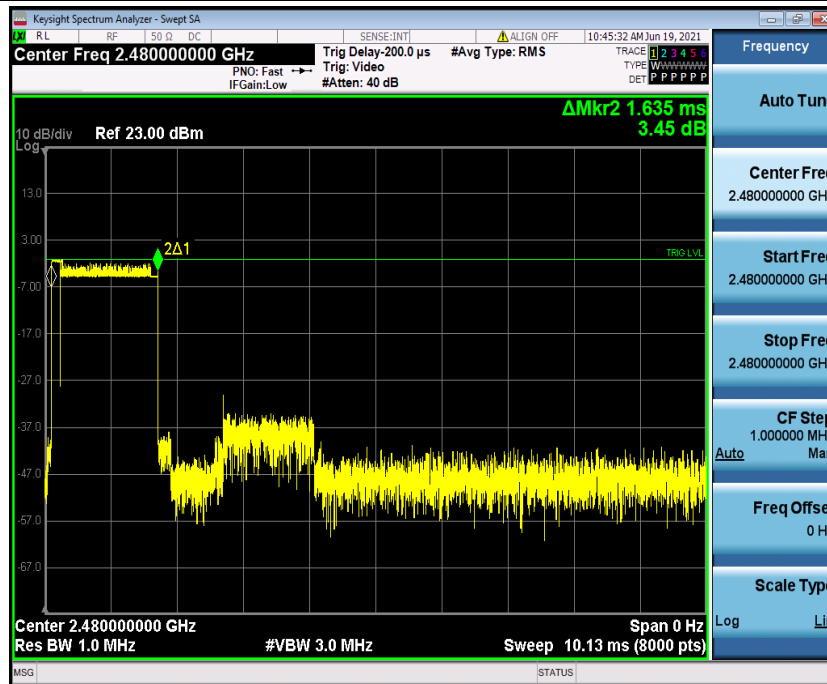
3DH3_Ant1_Hop_2480
