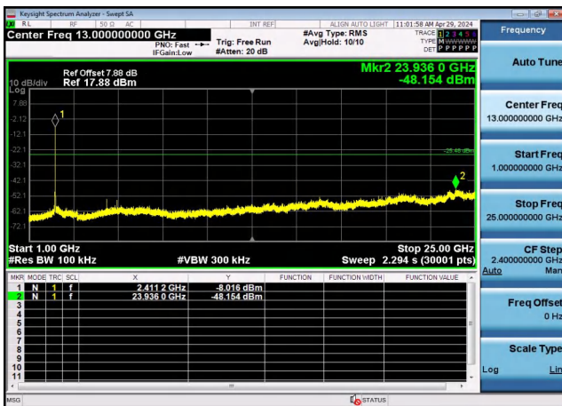
1GHz -25GHz
