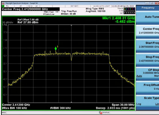
CH01
