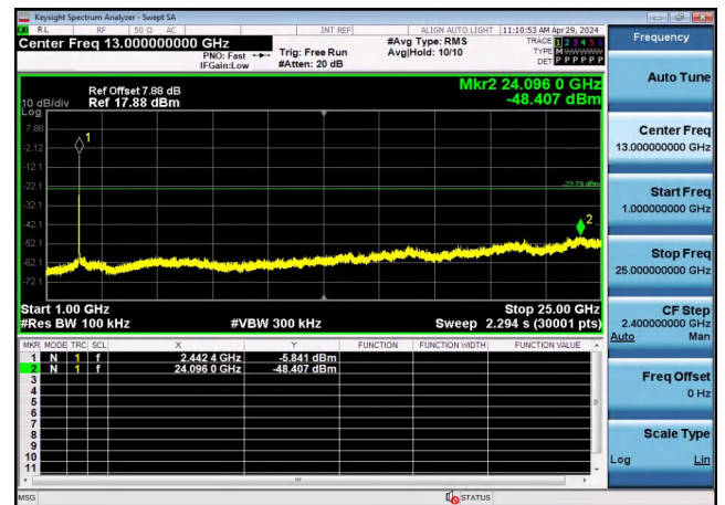
1GHz -25GHz
