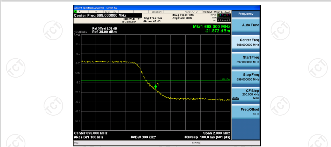
Band71-10MHz-QPSK-133172-50RB#0
